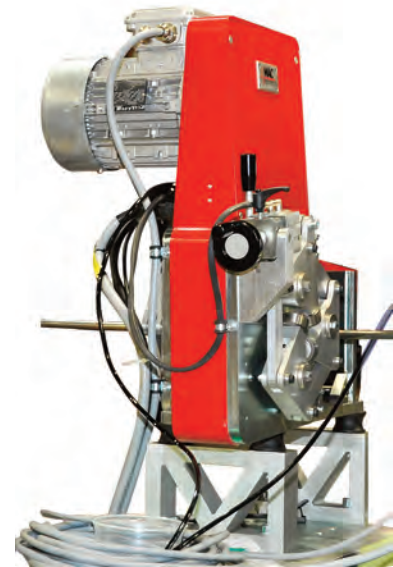
Der oben abgebildete Drehsondenprüfer wird mit Multimac-Elektronik zur Prüfung von Stangen oder Rohren mit einem Durchmesser von 3 mm bis 38,1 mm verwendet
