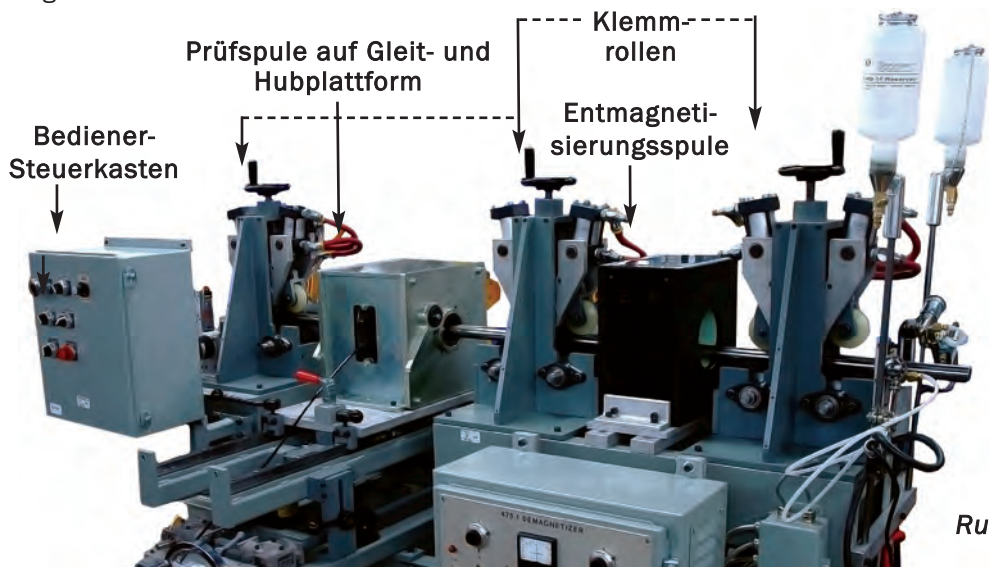
Der oben abgebildete Drehsondenprüfer wird mit Multimac-Elektronik zur Prüfung von Stangen oder Rohren mit einem Durchmesser von 3 mm bis 38,1 mm verwendet
